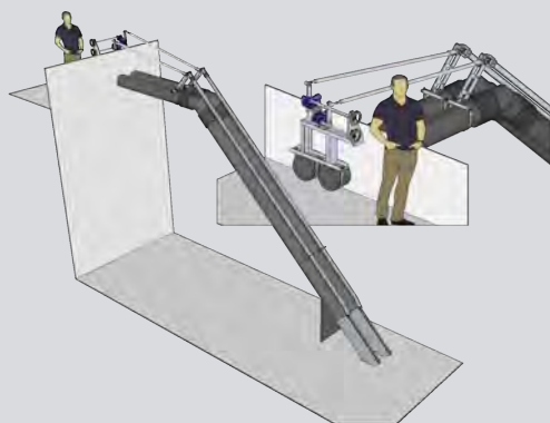
Røyrfilter utløpsrøyr
