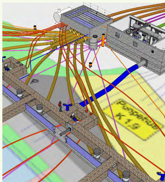
Tekning av rørsystem Rørsveis
